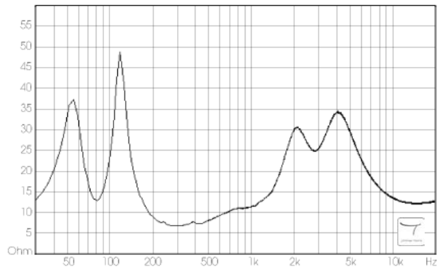
Impedanz
