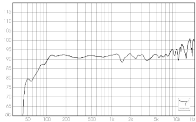
B&C 8NDL51 Hochton 3,5 db abgesenkt (3,9/10Ohm)
