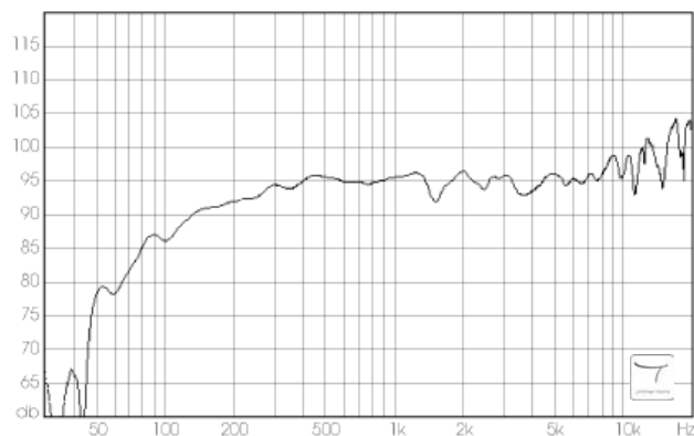
B&C 8NW51 und DE12 auf 106-Horn
